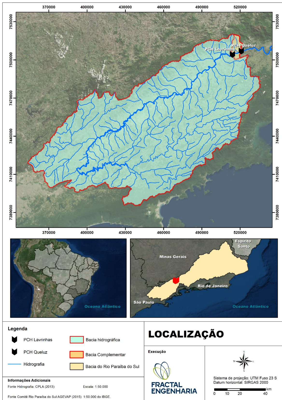
Figura 2. Mapa de Localização da PCH Lavrinhas.
